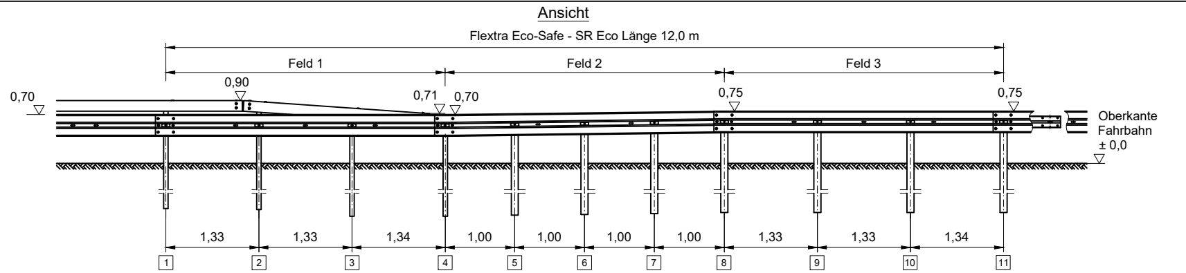
Ansicht nur Pfosten
