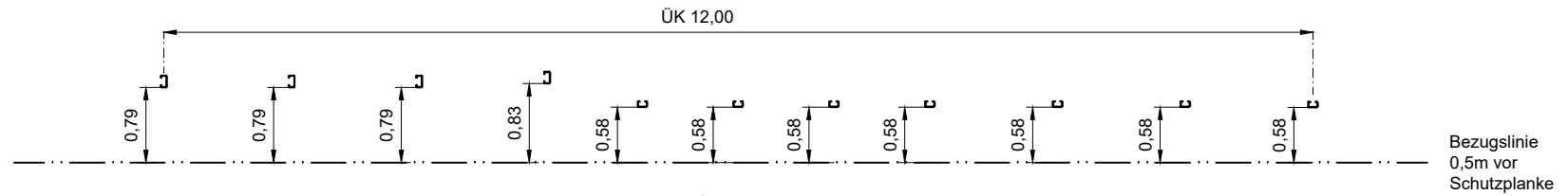
Draufsicht nur Pfosten
