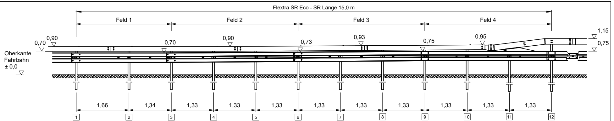
Ansicht nur Pfosten
