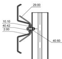
Pfostenverschraubung Profil B
