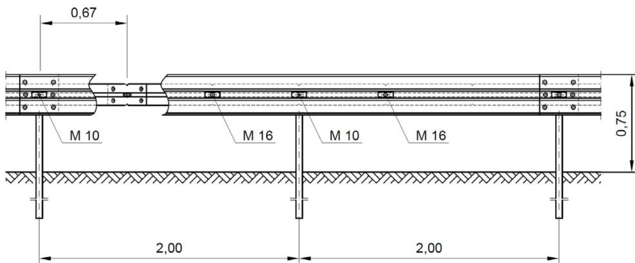
Pfostenverschraubung Profil B
