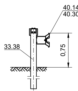
Schnitt D-D
