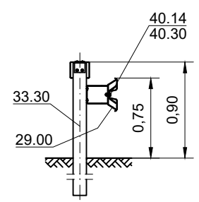
Schnitt C-C
