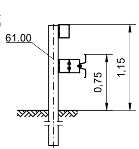
Schnitt A-A
