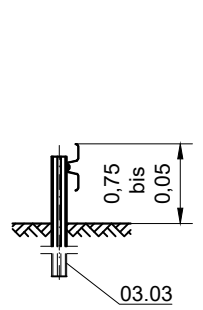
Schnitt F-F
