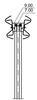
Schnitt A-A
