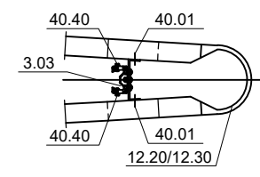
Einzelheit Z
