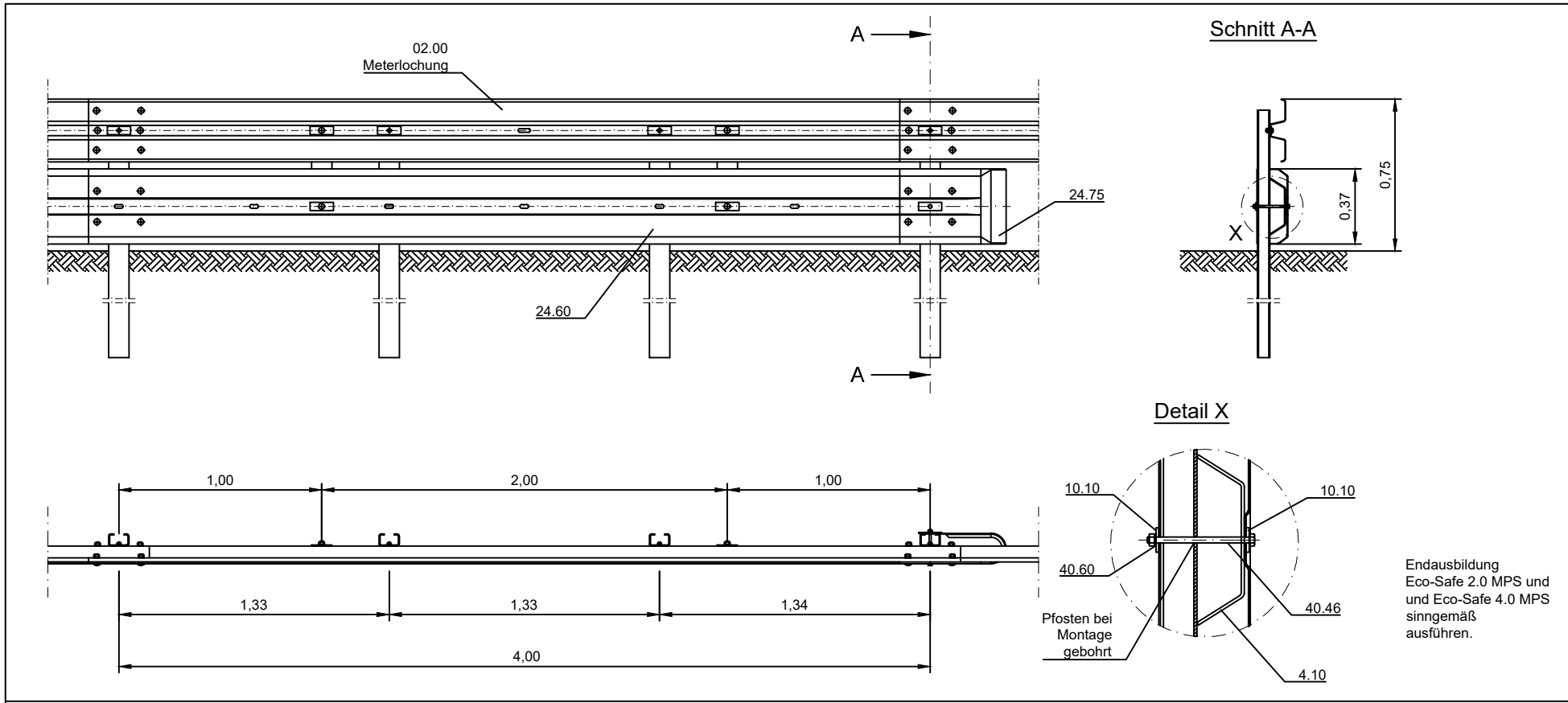
Alternative Endausbildung mit abgesenktem MPS- Unterfahrerschutzholm
