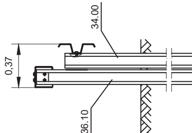
Schnitt B-B
