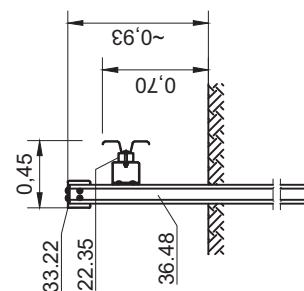
Pfosten 3
