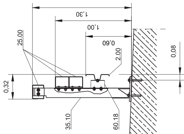
Schnitt A-A
