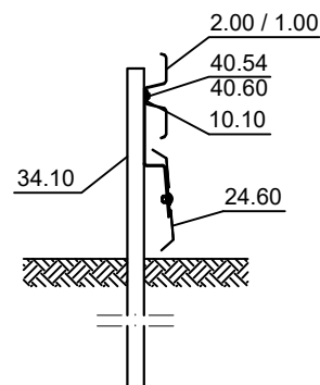
Schnitt C-C
