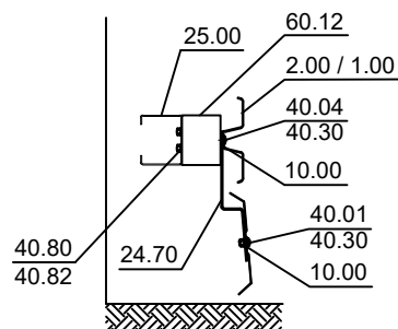
Schnitt A-A
