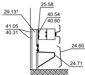
Schnitt B-B
