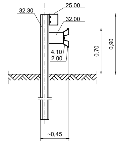
Schnitt A-A
